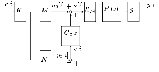
図5 制御器の実装
