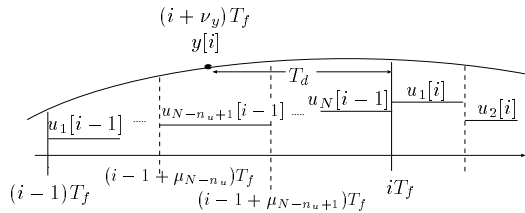
図7 むだ時間のタイムチャート
