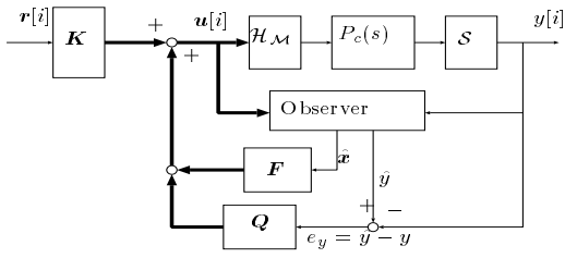
図4 2自由度制御系の基本構造
