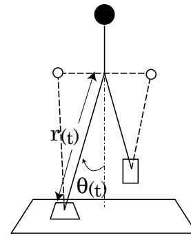
付図 1 前額面における歩行モデル
