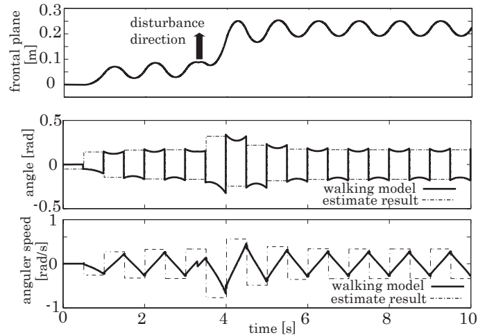
付図 2 歩行中の前額面での運動シミュレーション
