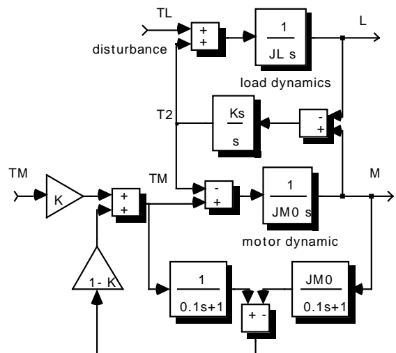
図7 共振比制御
