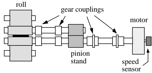
図 1 圧延機駆動系の構成
