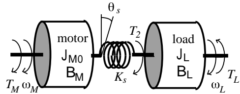
図 2 2 慣性系モデル
