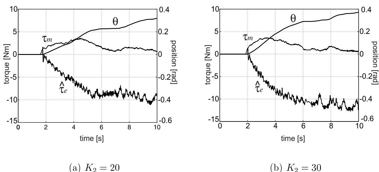
図 3.17: 剛性インピーダンスを加えた双方向インピーダンス制御によるパワーアシスト (ゴム 6 本)
