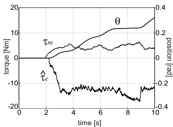
(b-1) D_e = 40, K_e = 400
