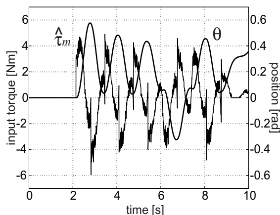
(d) M = 0.3, D = 2.0
