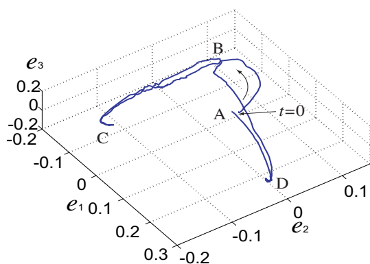
図 9.18: 3 次元固有空間上への投影軌跡
