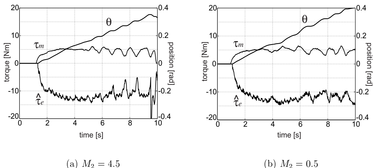
図 3.18: 双方向インピーダンス制御によるパワーアシストにおける慣性インピーダンスの効果 (段ボール)
