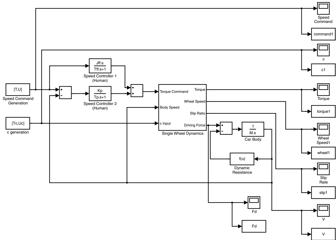
図 3.4: シミュレーション用の自動車の MATLAB モデル
