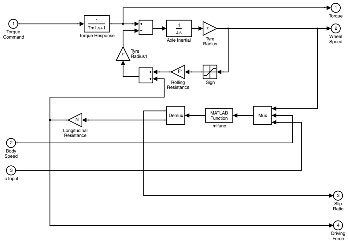
図 3.5: 車輪の MATLAB モデル
