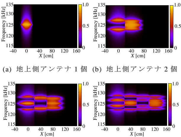
(a) 地上側アンテナ 1 個 (b) 地上側アンテナ 2 個 (c) 地上側アンテナ 3 個 (d) 地上側アンテナ 4 個 Fig. 7 効率の周波数特性 (クロスカップリングなし)
